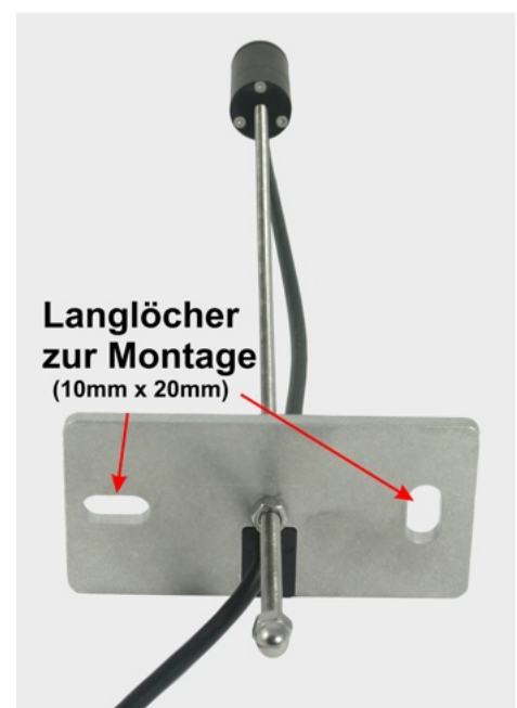
Bild 9 Mikrofonhalteplatte
